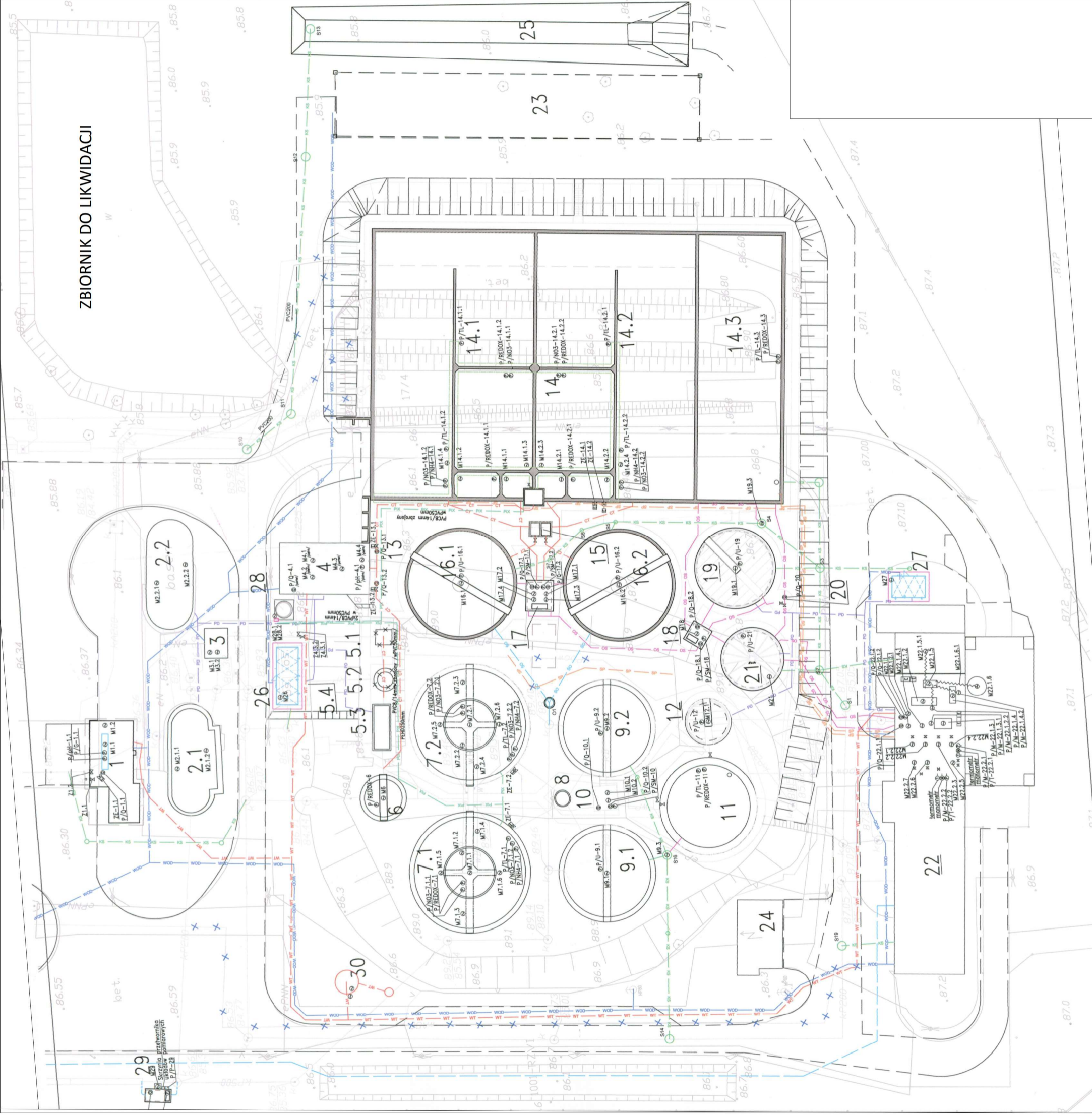
ZAL. 1 Schemat stanu istniejącego - Główne elementy oczyszczalni w Radziminie
